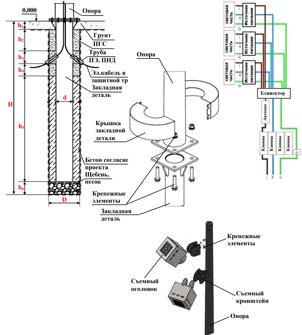
Рис.2 Схема монтажа и подключения светильника
