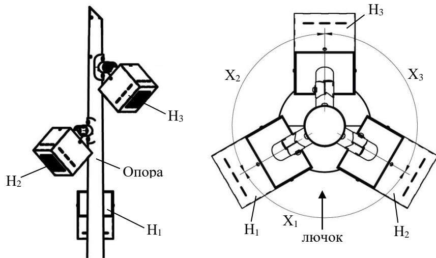
Высота расположения оголовка H_1 , H_2 , H_3 и угол разворота оголовков X_1 , X_2 , X_3 – согласно заказу
