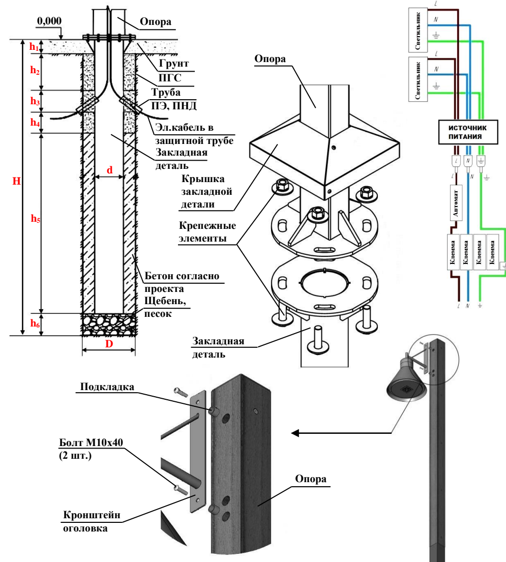
Рис.1 Схема монтажа и подключения светильника
